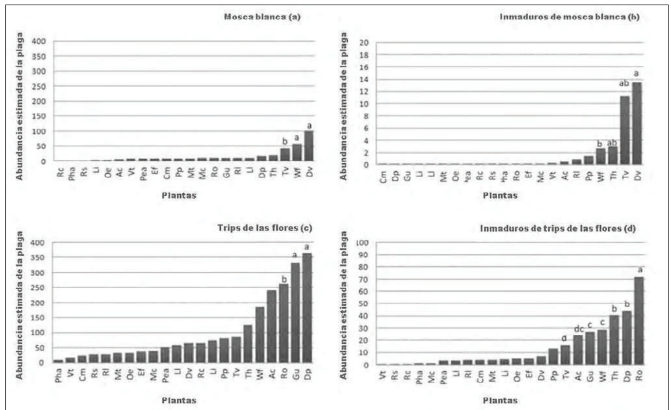
Figura 2. Valor estimado de la abundancia por planta arbustiva de adultos+estados inmaduros de mosca blanca (a), estados inmaduros de mosca blanca (b), adultos+estados inmaduros de trips (c) y estados inmaduros de trips (d). Separación de medias mediante test de Tuckey. Las letras pequeñas denotan diferencias significativas entre plantas arbustivas ( p < 0.05 ). Las diferencias significativas solo fueron mostradas cuando la abundancia estimada fue mayor o igual a la media del valor estimado. Consultar código de las plantas en Tabla 1.
